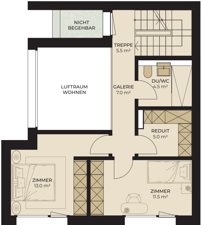
OBERGESCHOSS
