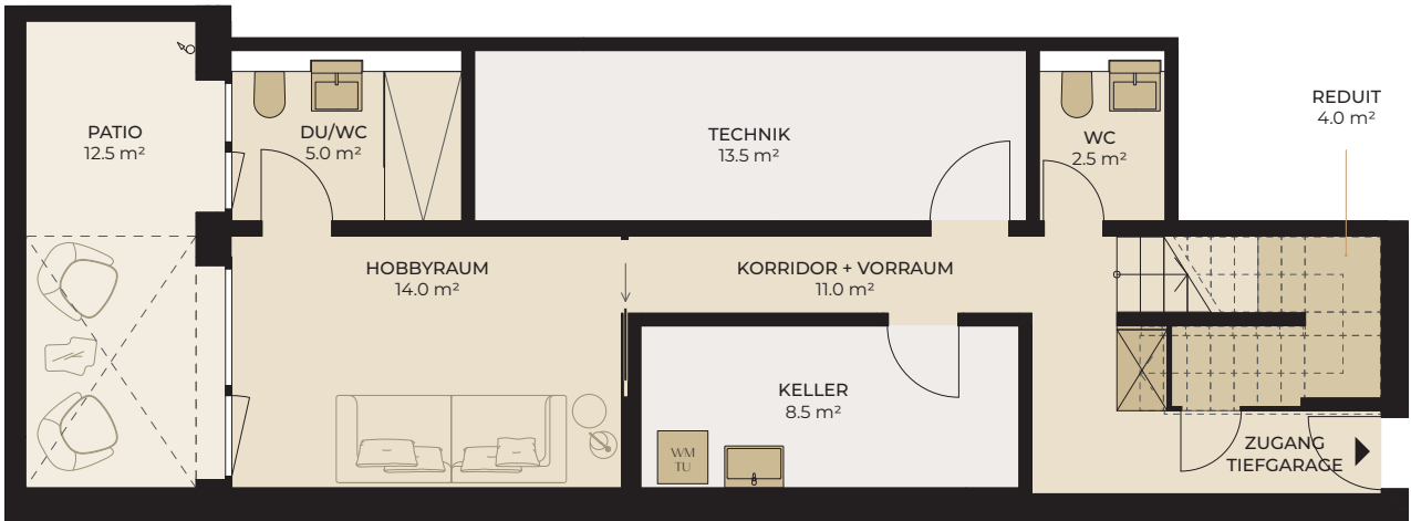
UNTERGESCHOSS
