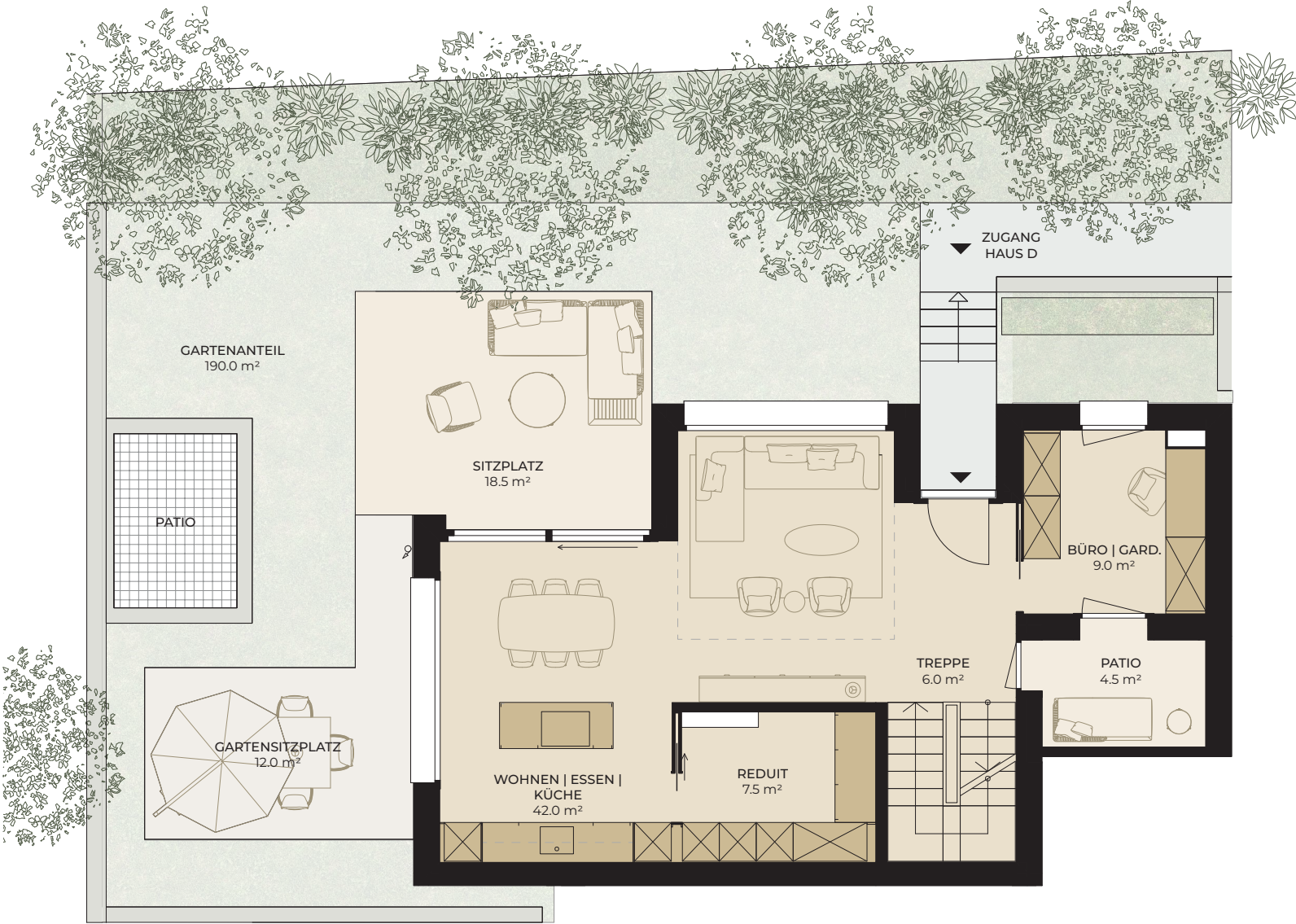
ERDGESCHOSS
