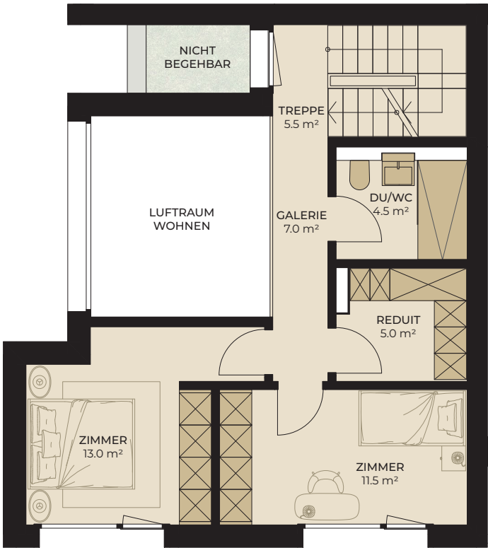
OBERGESCHOSS
